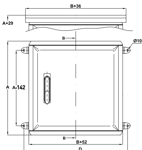
Dimensiones (mm)
