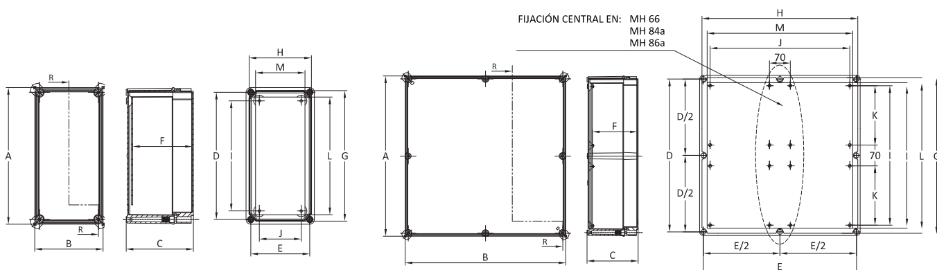
Dimensiones cajas (mm)
